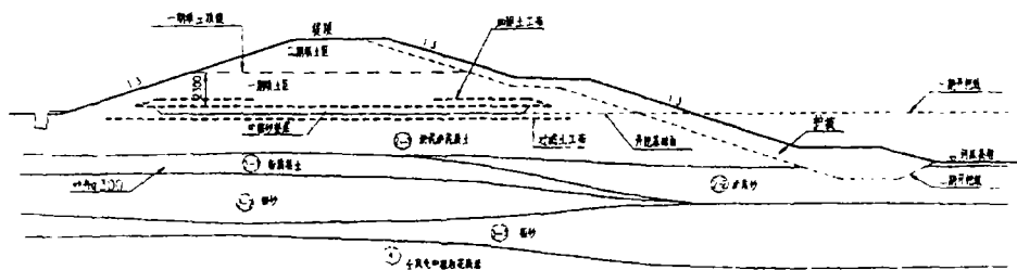
图2 治理深圳河第二期工程加固土工布施工示意图
