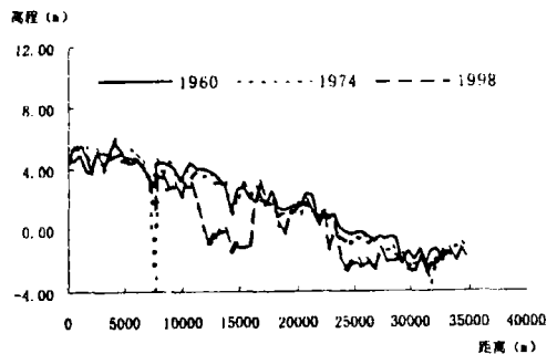
图2f 东溪河道纵剖面平均河底高程
