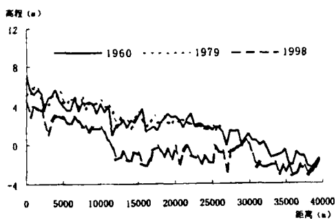
图2e 西溪河道纵剖面平均河底高程
