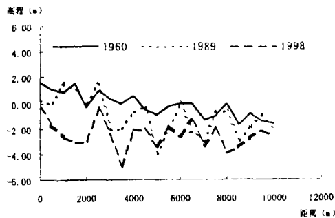
图2d 南溪河道纵剖面平均河底高程
