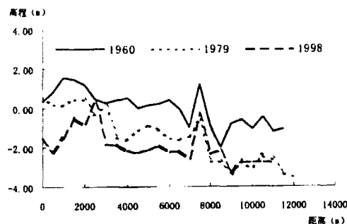
图2c 梅溪河道平均河底高程
