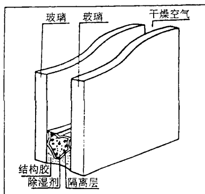
图1 中空玻璃
