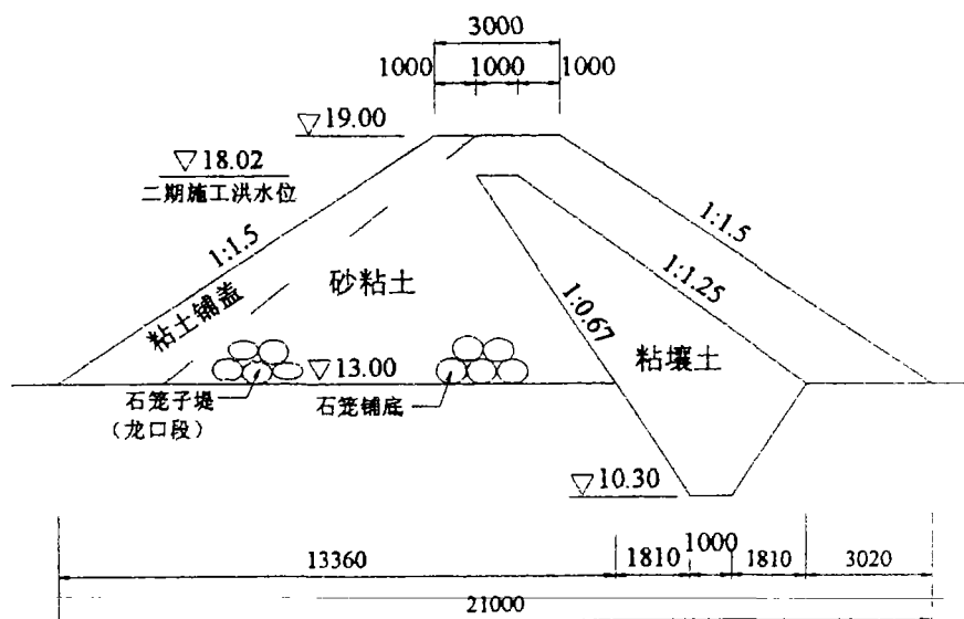
图2 二期上游围堰典型断面
