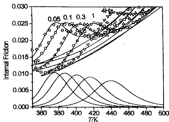
图3 P_2 内耗峰的实验数据与拟合曲线
