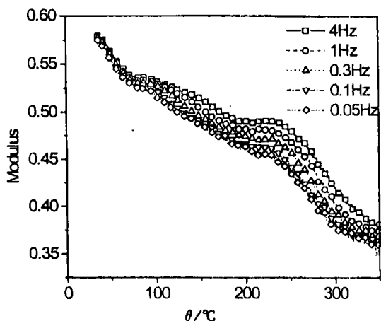
图2 模量温度曲线
