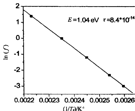
图4 \ln(f) 与 1/T_p 关系
