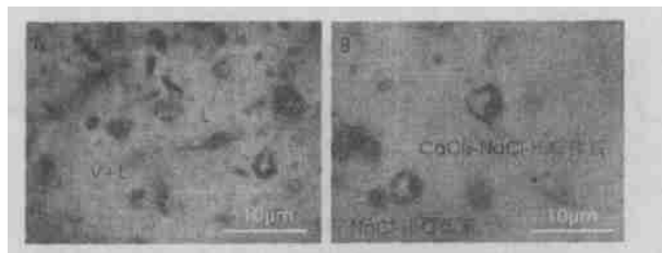
图4 铂多金属矿流体包裹体中纯液相和气液二相共存(a)和高盐度CaCl 2 -NaCl-H 2 O体系和低盐度NaCl-H 2 O体系共存(b)现象
