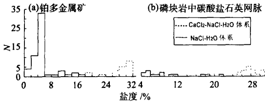
图 3 流体包裹体的盐度分布直方图
