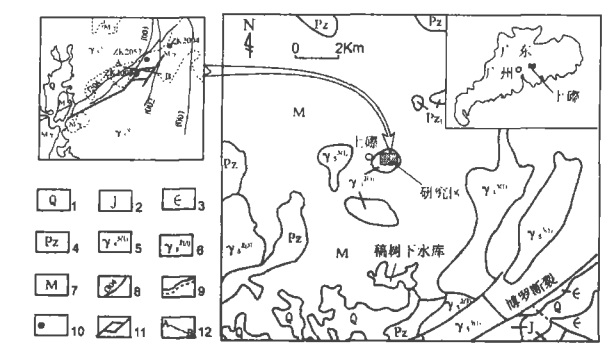
图 1 研究区区域地质简图 (据 1/20 万惠州幅地质图改编), 左上方小图为研究区地质简图 Fig. 1 Schematic geological map of study district 1 第四系; 2 侏罗系; 3 寒武系; 4 古生界 (未分); 5 燕山三期花岗岩; 6 燕山二期花岗岩; 7 混合岩; 8 断裂; 9 实 推测地质界线; 10 钻孔; 11 探洞; 12 剖面线
