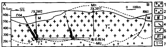
图 3 复式岩体示意剖面 (剖面位置见图 1 左上方小图) Fig. 3 Schematic section of the composite granite body 1 燕山早期花岗岩; 2 燕山晚期花岗岩; 3 混合岩; 4 石英-萤石脉; 5 断裂; 6 重熔界面; 7 钻孔
