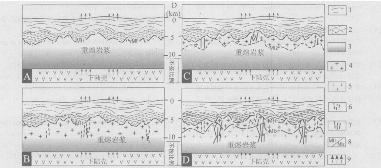
图 5 研究区内各类岩石的关系及成因模型 (据文献 [16] 改编)
