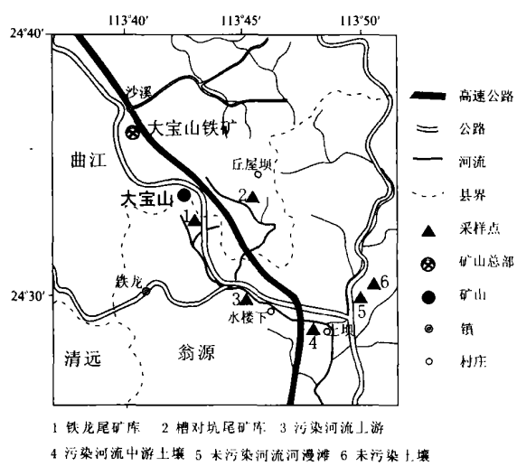
图 1 大宝山地理位置图 Fig 1 Location of the Dabaoshan polymetallic ore deposit
