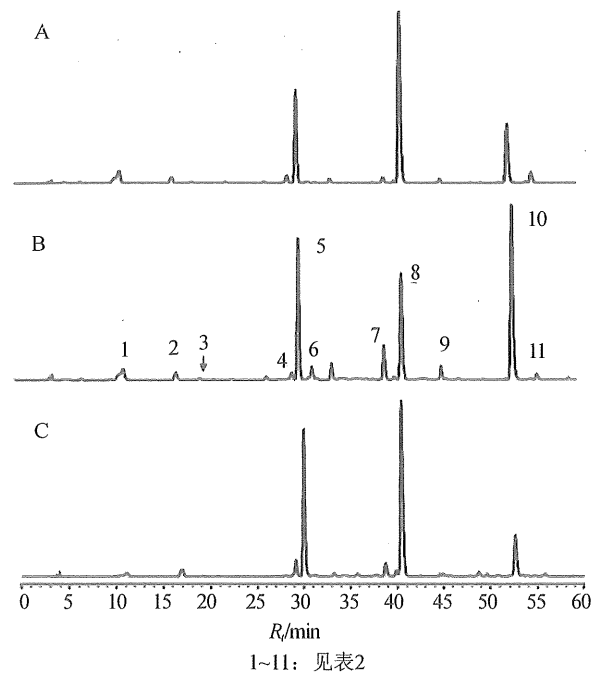
图 2 英红 1 号 (A)、英红 9 号 (B) 和祁门茶树 (C) 芽叶的 HPLC 色谱图 (275 nm)
