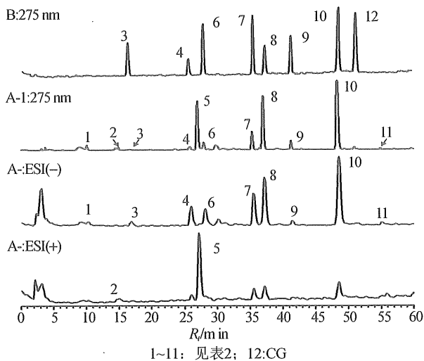
图 1 英红 9 号芽叶 (A-1 ~ A-3) 和儿茶素混合对照品 (B) 的 HPLC-UV-MS 色谱图
