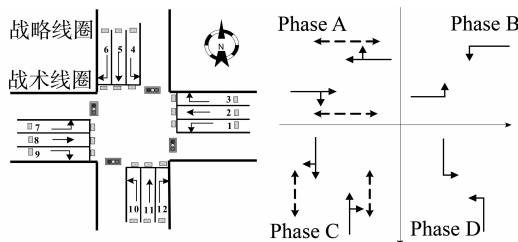
图 5 单交叉口模型示意图
