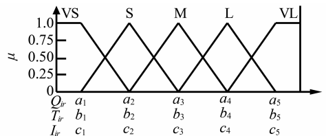
图 3 隶属参数编码原理示意图
