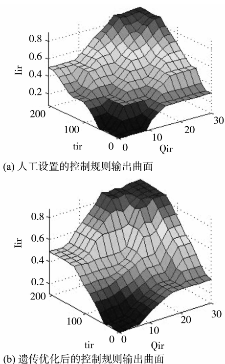
图 9 红灯紧迫度判定模块的控制规则输出曲面
