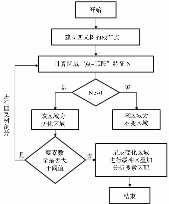
图 3 基于四叉树的变化捕捉算法流程图
