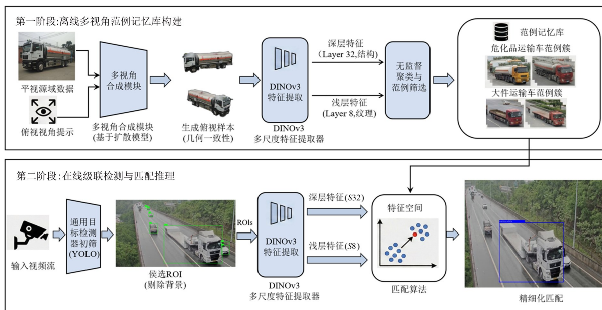
图2 总体框架图
